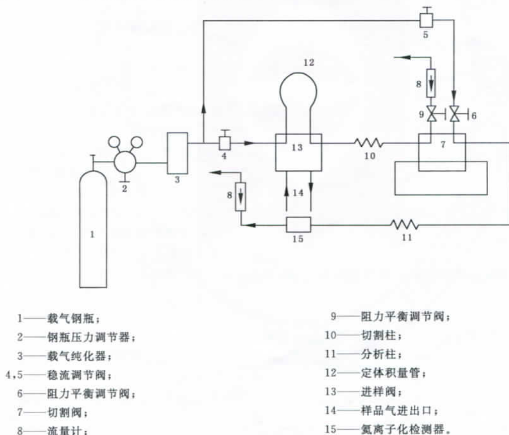
图 A.1 气路流程示意图
